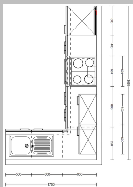
Wandansicht 2
